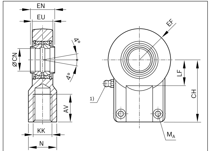
1) Engrasador cónico, forma A según DIN 71412
