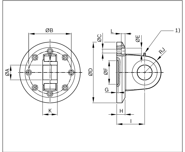
1) Engrasador cónico, forma A según DIN 71412
