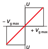
HS/HS4 (RS 92076) Variador hidráulico de la cilindrada (servoválvula/válvula proporcional)
