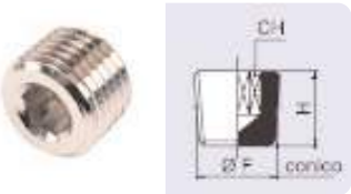
POA: TAPÓN ALLEN CONICO. M.
