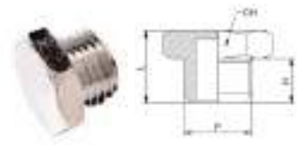
PO-G: TAPÓN CILÍNDRICO M.
